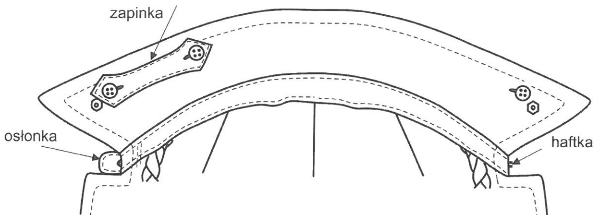
Rysunek 8. Kołnierz - spód
